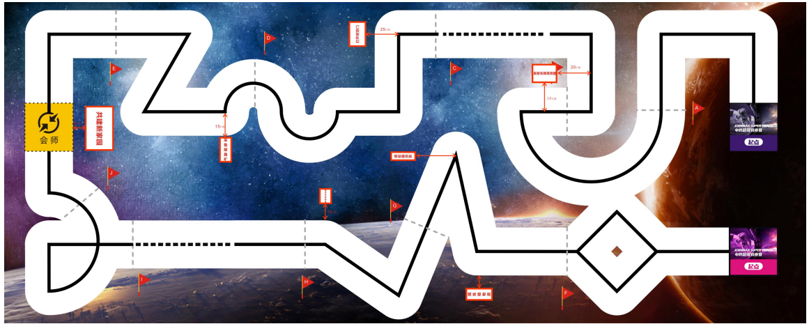
图 1 2021 江西省赛超级轨迹场地布置平面示意图
